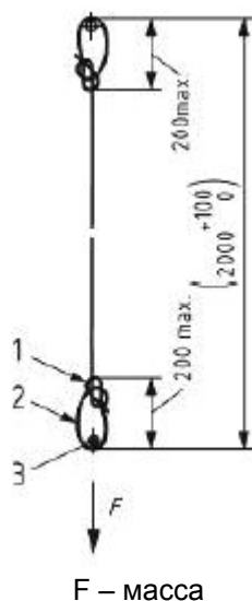
Рисунок 6 - Испытательная стропа для проверки прочности динамической нагрузкой
