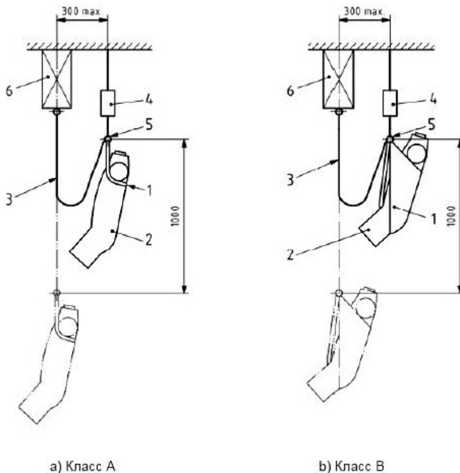
Рисунок 7 - Проверка прочности спасательных петель классов А и В динамической нагрузкой
