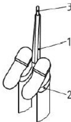
Рисунок 3 - Пример спасательной петли класса С в положении для спасания
