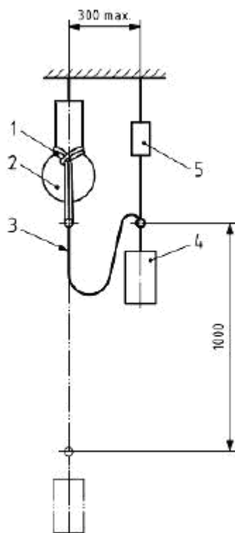
Рисунок 8 - Проверка прочности спасательных петель класса С динамической нагрузкой
