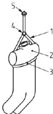
Рисунок 1 - Пример спасательной петли класса А
