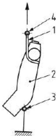
Рисунок 9 - Проверка прочности спасательных петель класса А статической нагрузкой
