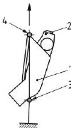
Рисунок 10 - Проверка прочности спасательных петель класса В статической нагрузкой
