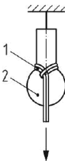
1 - спасательная петля; 2 - испытательная форма (Вернуться к содержанию)
